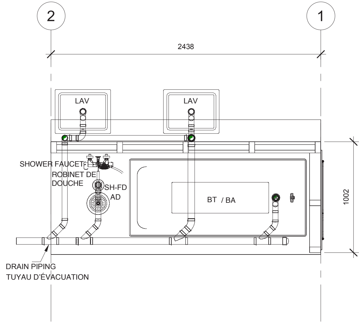
2 TOP VIEW / VUE DE PLAN 1 : 20
