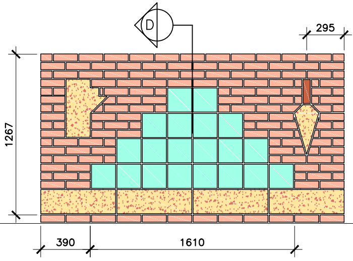
ELEVATION ÉLÉVATION
