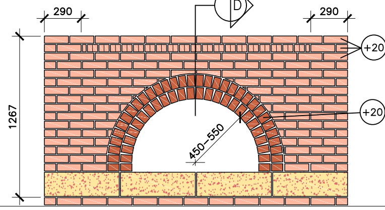
ELEVATION ÉLÉVATION
