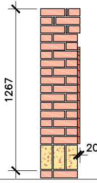
ELEVATION ÉLÉVATION
